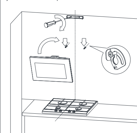
Rys. 7 Zawieszanie okapu.
