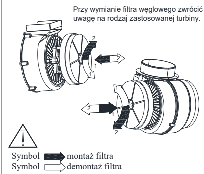
Rys.11 Wymiana filtra węglowego.
