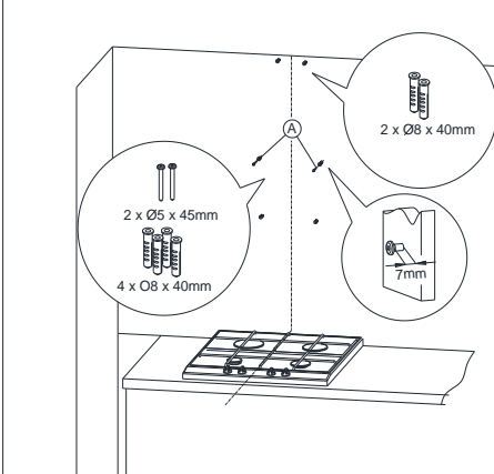
Rys. 7 Zawieszanie okapu.
