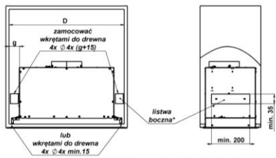
Rys. 6b Mocowanie okapu – wersja mocowania bocznego
