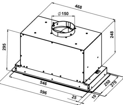
Rys. 2 Rysunek gabarytowy
