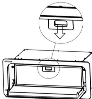
Rys. 5 Demontaż filtra przeciwłuszczowego
