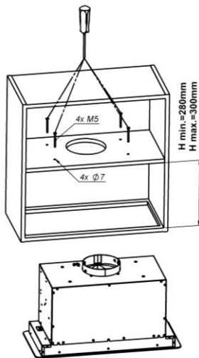
Rys. 6a Montaż okapu – wersja mocowania górnego
