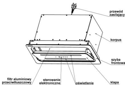
Rys. 1 Rysunek poglądowy okapu
