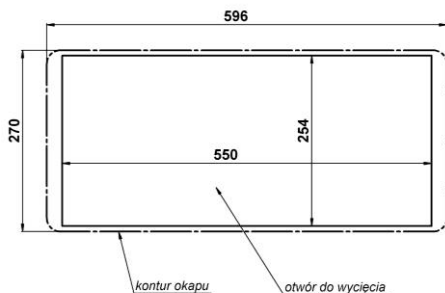
Rys. 4 Przygotowanie szafki
