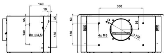
Rys. 6c Otwory montażowe
