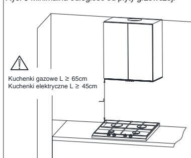
Rys. 3 Minimalna odległość od płyty grzewczej.
