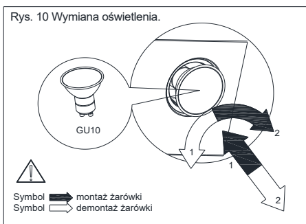
Rys. 10 Wymiana oświetlenia.
