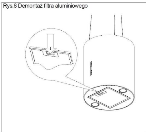
Rys.8 Demontaż filtra aluminiowego
