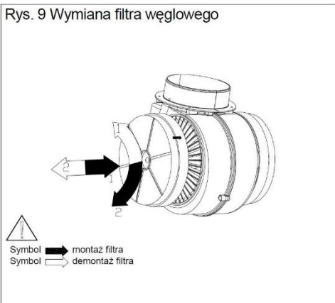
Rys. 9 Wymiana filtra węglowego
